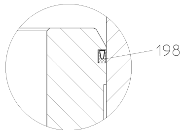
Рис. 24: Разгрузочное уплотнение, кольцо Variseal, фиг. 0.1 (АТО) – выноска Z
