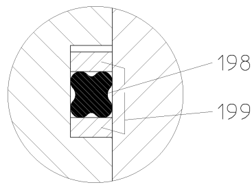
Рис. 23: Разгрузочное уплотнение, кольцо квадратного сечения – деталь Z
