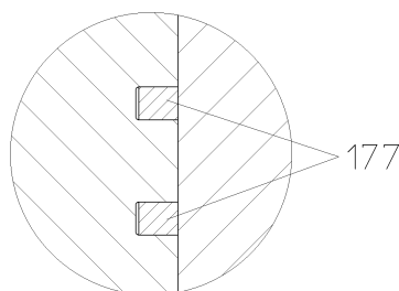
Рис. 22: Разгрузочное уплотнение, поршневые кольца – деталь Z
