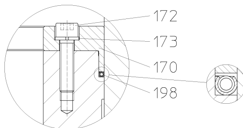
Рис. 26: Разгрузочное уплотнение, С-образное кольцо, фиг. 0.1 (АТО) – выноска Z
