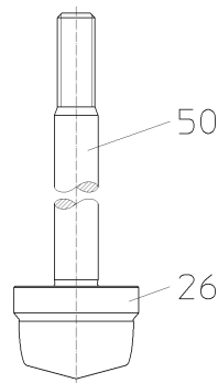
Рис. 21: Крепление плунжер - шток, стандарт
