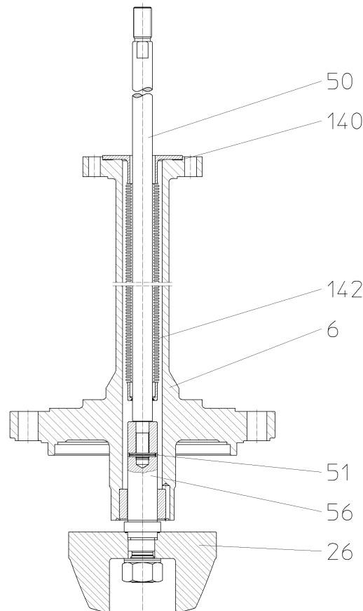
Рис. 19: Крепление плунжер - шток, сильфон
