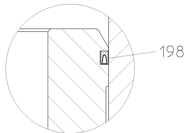
Рис. 25: Разгрузочное уплотнение, кольцо Variseal, фиг. 0.2 (АТС) – выноска Z
