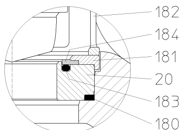
Рис. 28: Мягкое уплотнение, плоское уплотнение и кольцо круглого сечения – деталь Y
