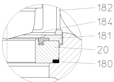
Рис. 29: Мягкое уплотнение, трапецеидальное кольцо – деталь Y
