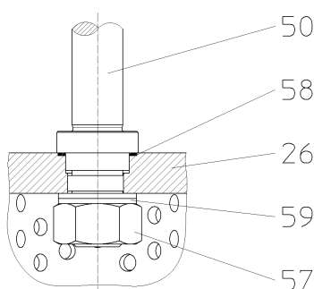
Рис. 18: Крепление плунжер - шток, стандарт
