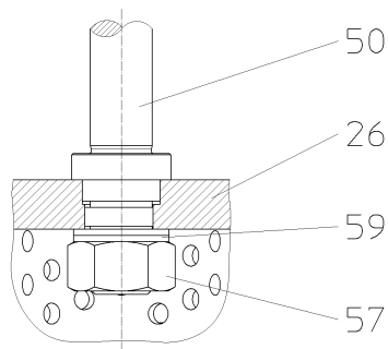
Рис. 20: Крепление плунжер - шток, разгрузка давления
