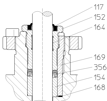
Рис. 17: Уплотнение Variseal
