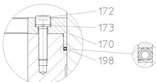
Рис. 27: Разгрузочное уплотнение, С-образное кольцо, фиг. 0.2 (АТС) – выноска Z
