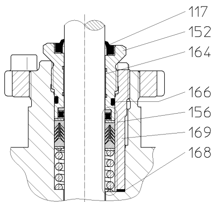
Рис. 13: V-образные манжеты
